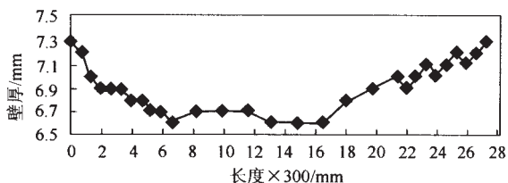
图3 在钢管长度方向的壁厚变化
