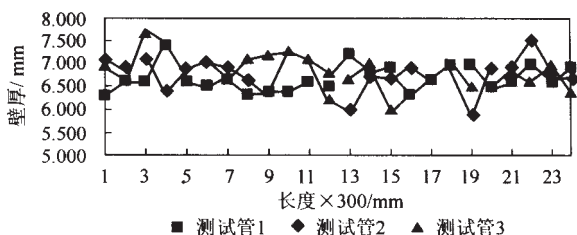
图1 低温(760℃)定径时对钢管壁厚的影响
