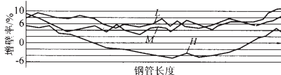
图2 在不同速度系列下增壁率沿长度方向的变化规律
